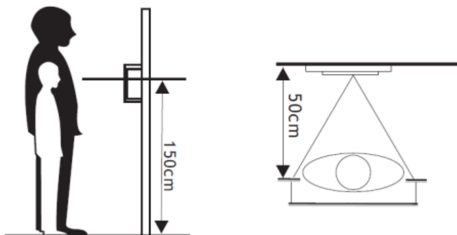
Пример установки вызывной панели на стену
