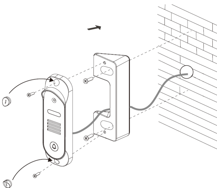
Пример установки вызывной панели на стену
