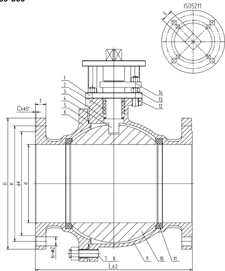
Рисунок 3 – Детализовка и размеры для Ду250-300
