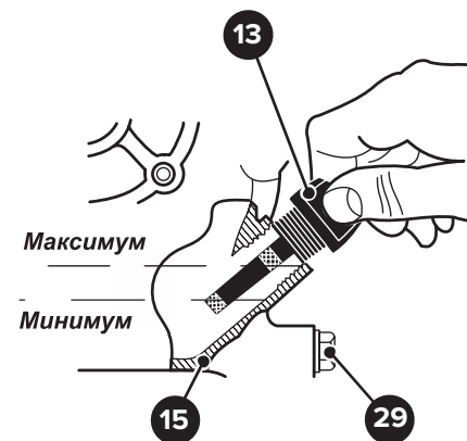
13. Пробка (для заливки масла)
