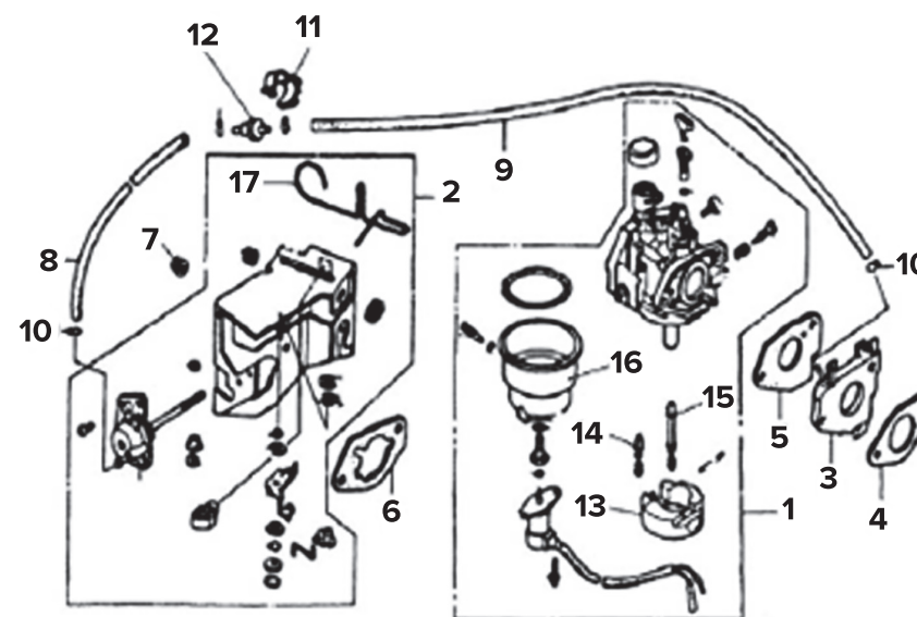
Схема сборки № 8
