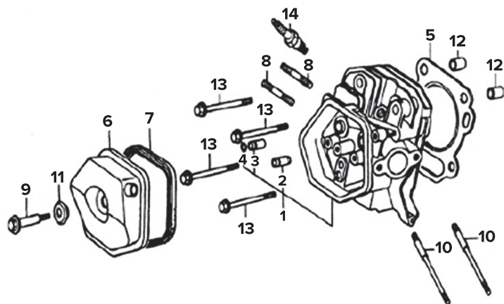
Схема сборки № 1
