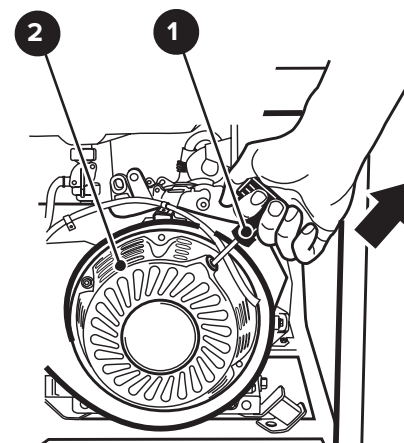
2. Ручной стартер
