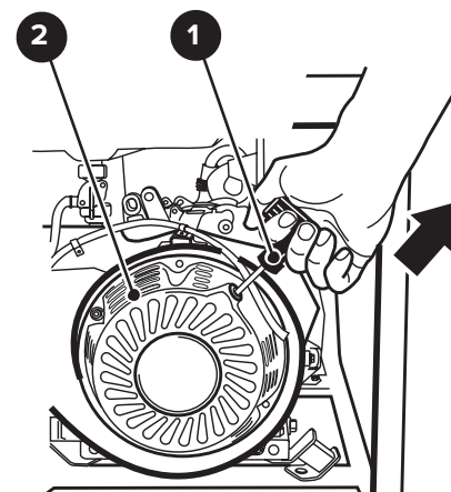
2. Ручной стартер
