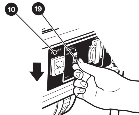
19. Автомат защиты от перегрузки
