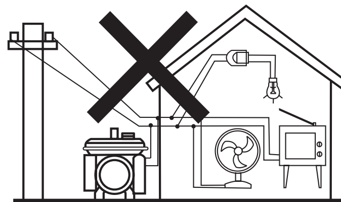
Рисунок 14 — Неправильное подключение генератора к промышленной электрической сети — без блокировок
