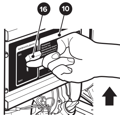
10. Панель управления (выключения) цепи зажигания двигателя 16. Клавиша (выключатель) включения
