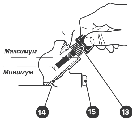
13. Пробка (для заливки масла) 14. Двигатель
