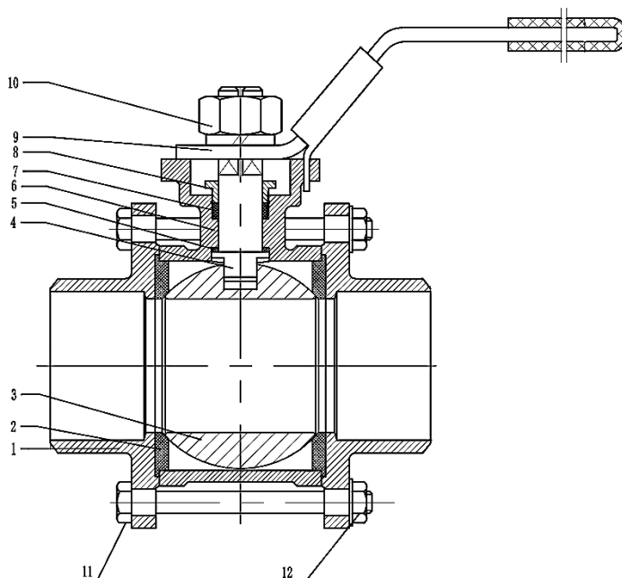
Рисунок 2 - Деталировка
