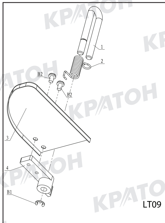
Схема сборки № 10. Ограждение защитное LT09
