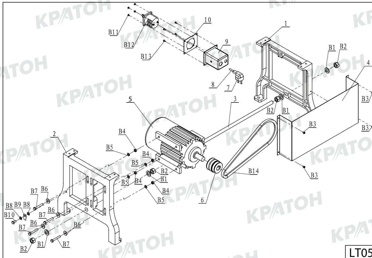
Схема сборки № 6. Основание LT05
