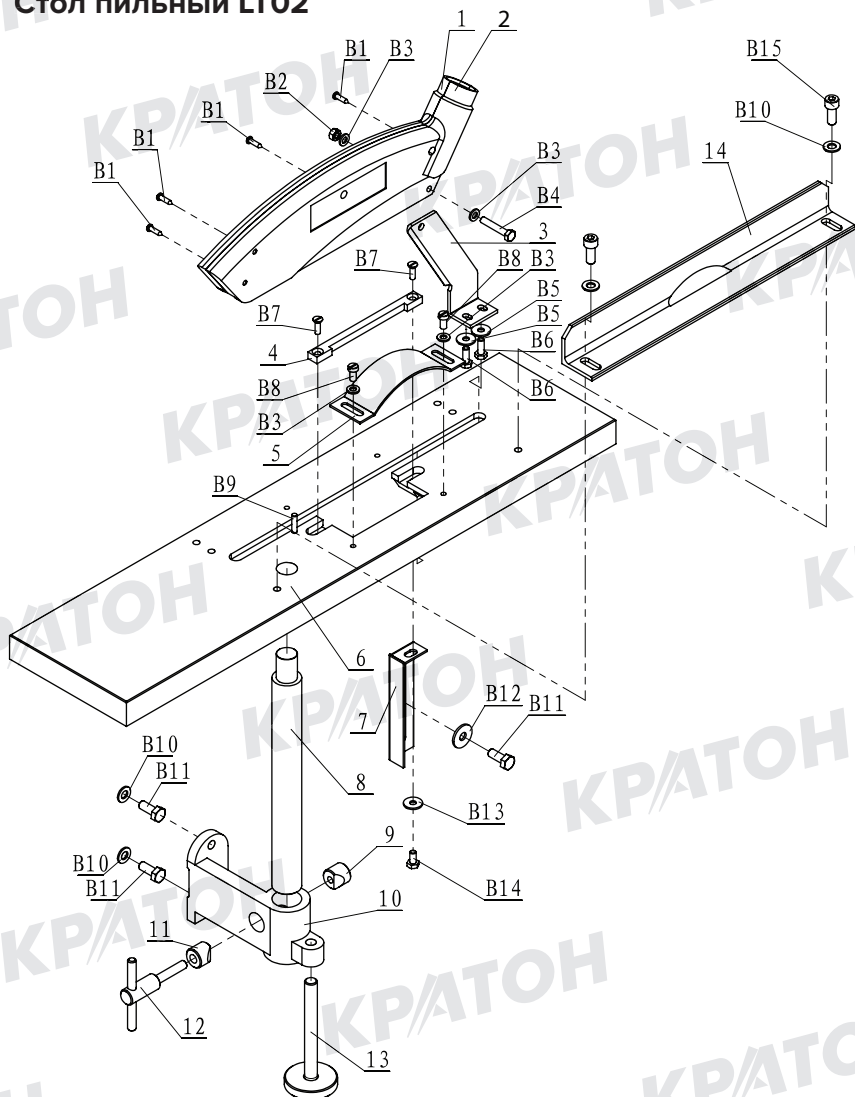
Схема сборки № 3. Стол пильный LT02
