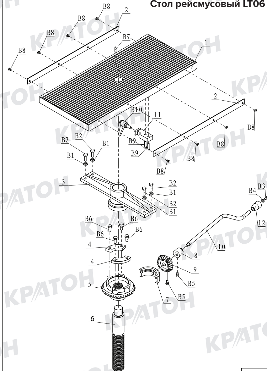
Схема сборки № 7. Стол рейсмусовый LT06
