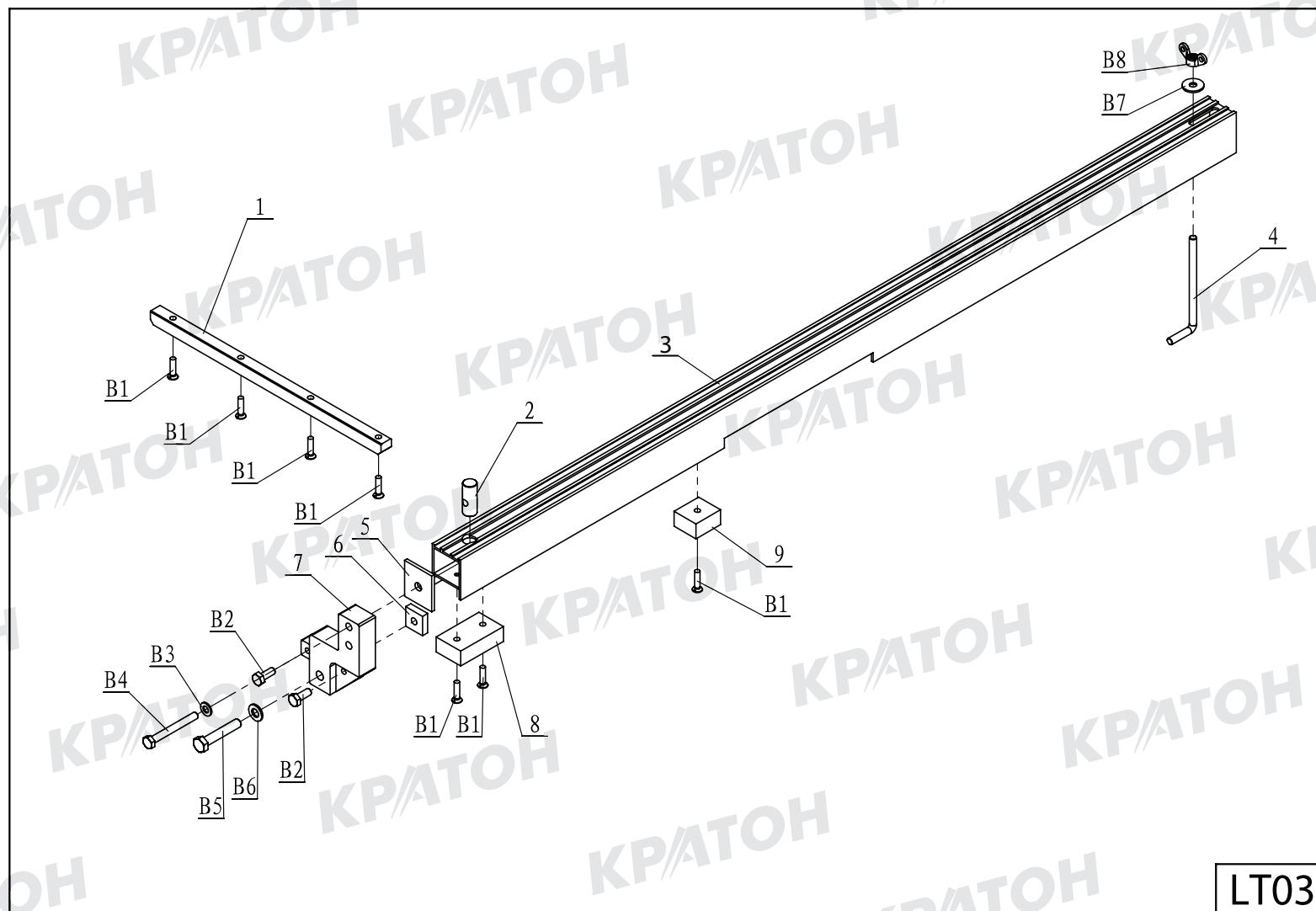
Схема сборки № 4. Линейка направляющая LT03
