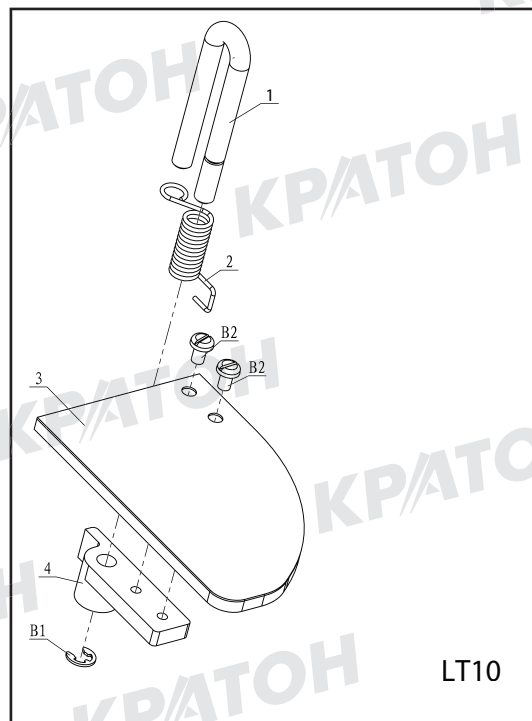
Схема сборки № 11. Ограждение защитное LT10
