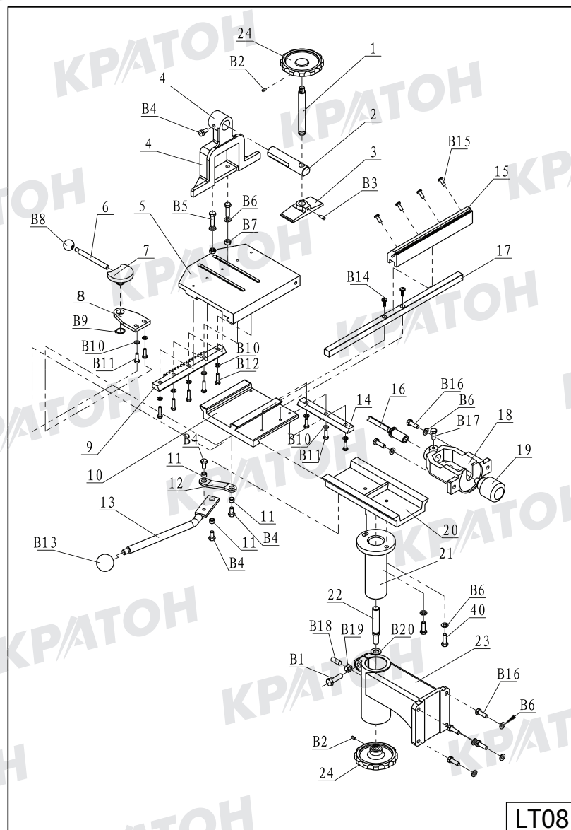
Схема сборки № 9. Суппорт фрезерный LT08
