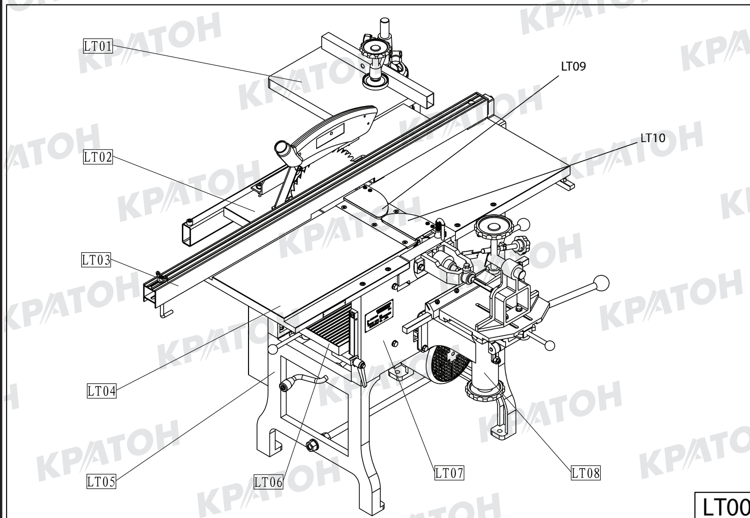
Схема сборки № 1. Общий вид LT00
