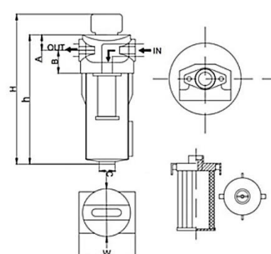
Фильтр CJ
