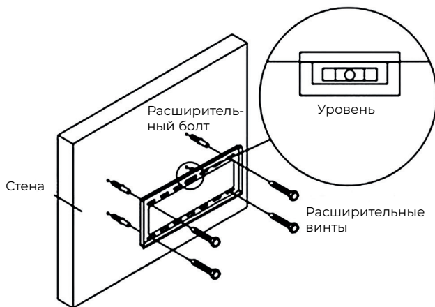
Рис.2. Схематичная установка.
