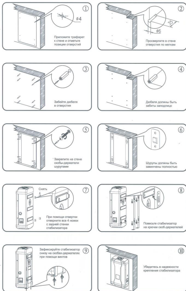
Монтажный трафарет Рис. 3
