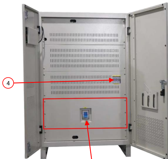
Рис. 1 Модели 100кВА-200кВА
