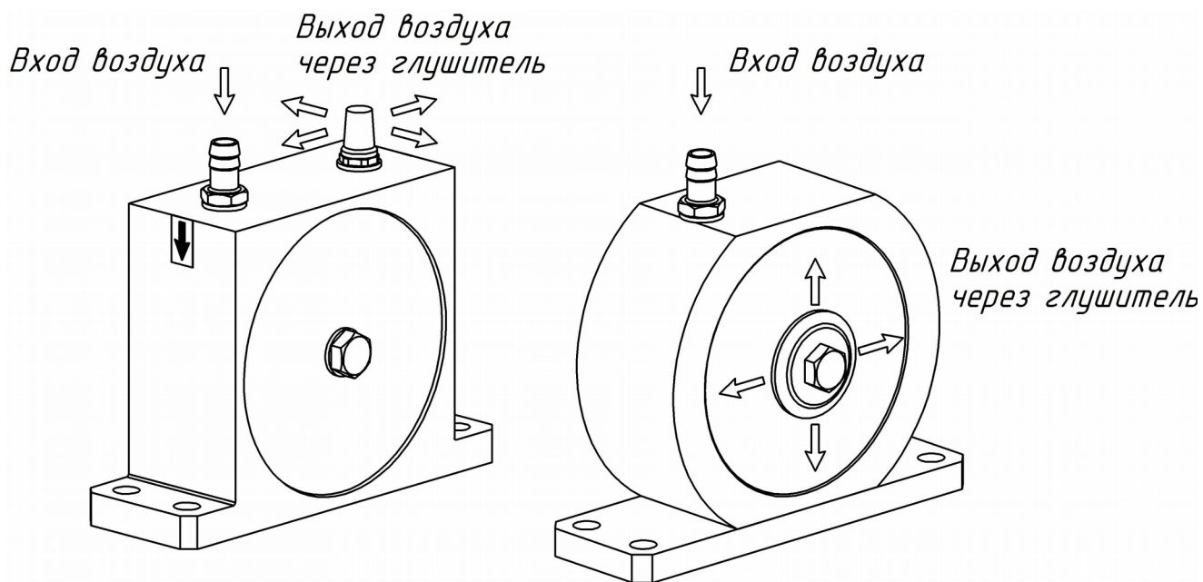
Рисунок 4. Схема подачи и отвода сжатого воздуха
