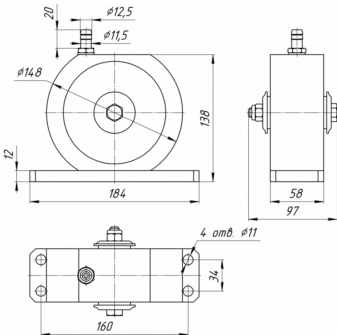
Рисунок 3. Вибратор ИВШ-41
