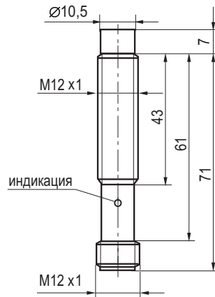
Габаритный чертеж
