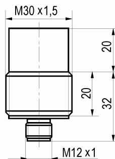
Габаритный чертеж
