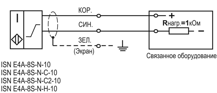
Схема подключения к оборудованию
