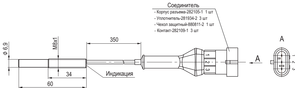
Габаритный чертеж
