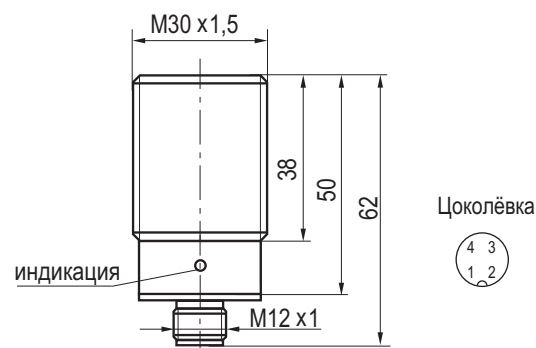
Габаритный чертеж
