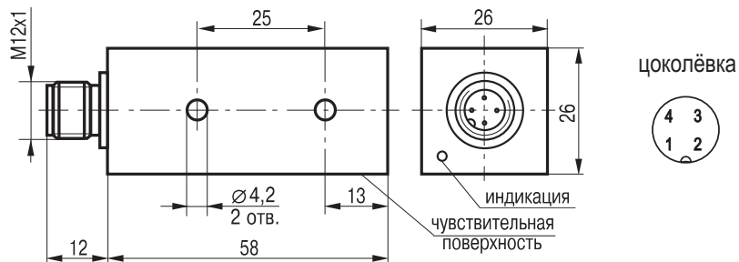
Габаритный чертеж
