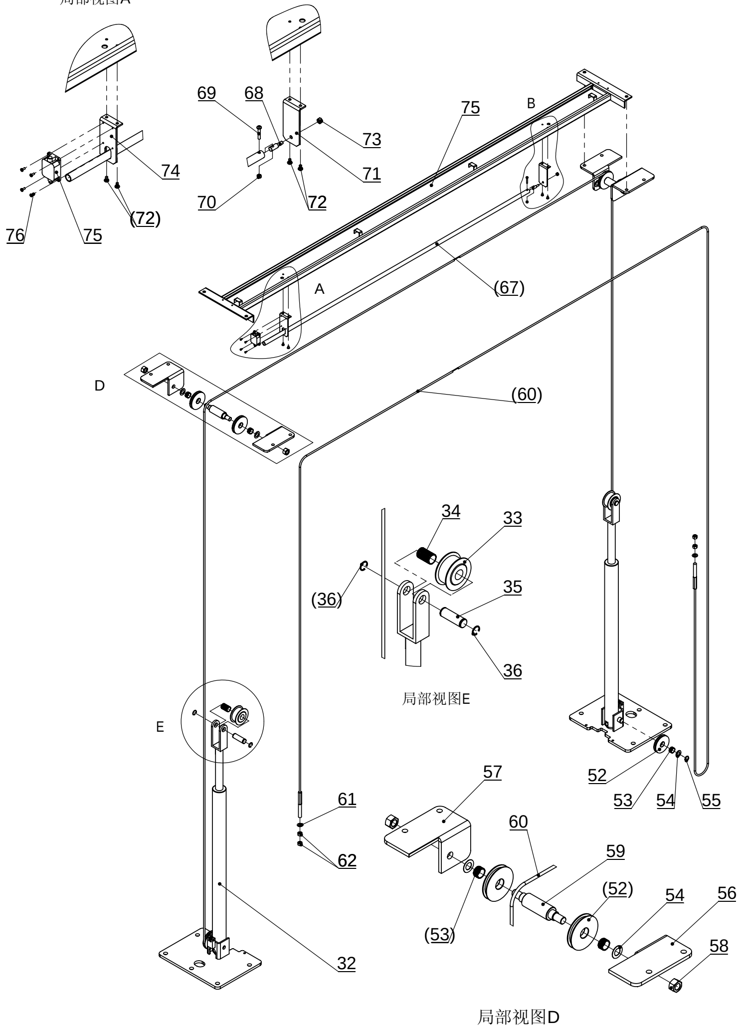
局部视图A
