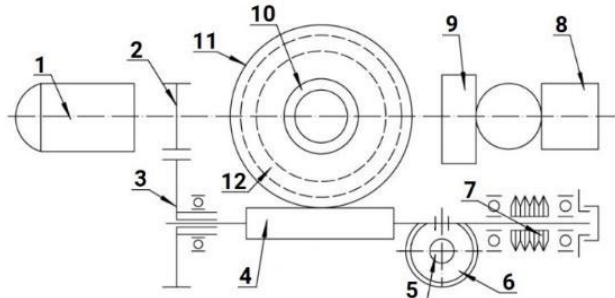
Рисунок 3 – Элементы электропривода
