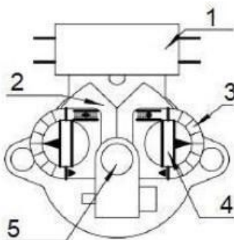
Рисунок 4 – Элементы механизма управления крутящим моментом
