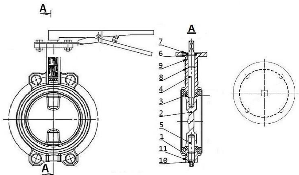
Рисунок 1. Деталировка
