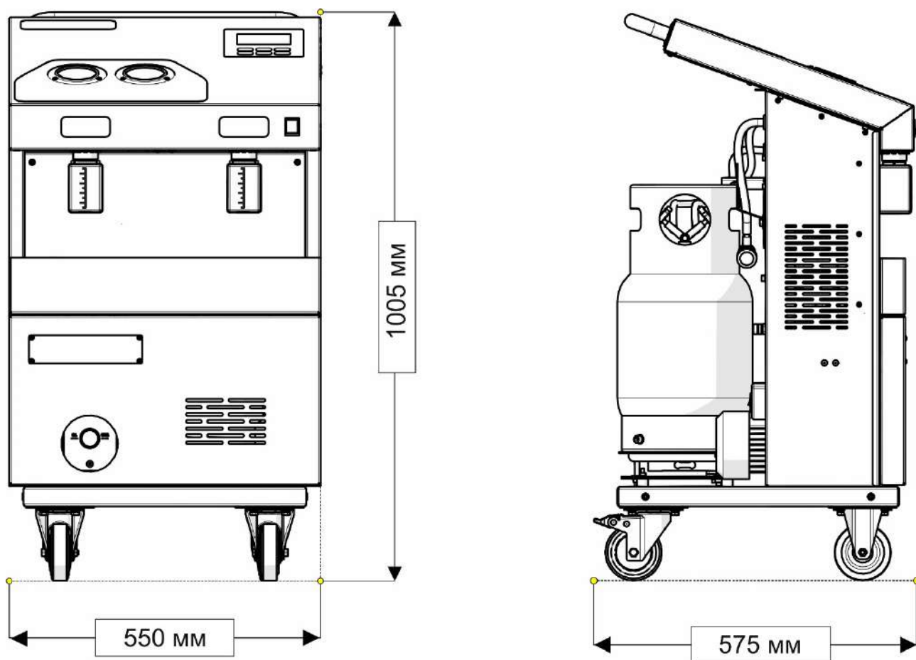
Рис. 1 Общий вид установки
