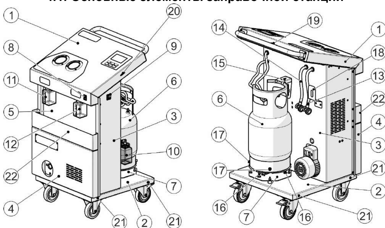
Рис. 2 Основные элементы станции ODA-450
