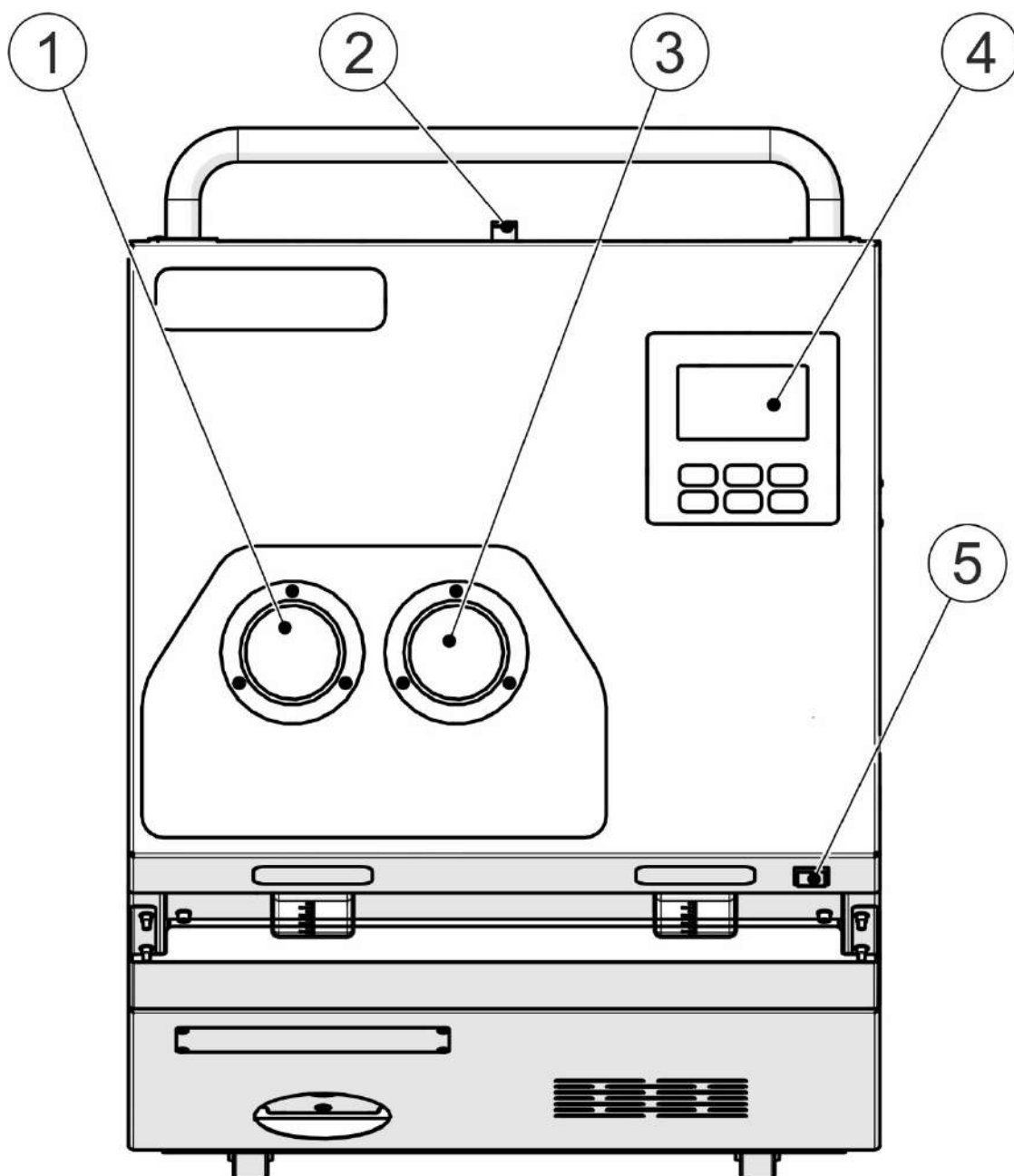
Рис. 3 Лицевая панель станции.
