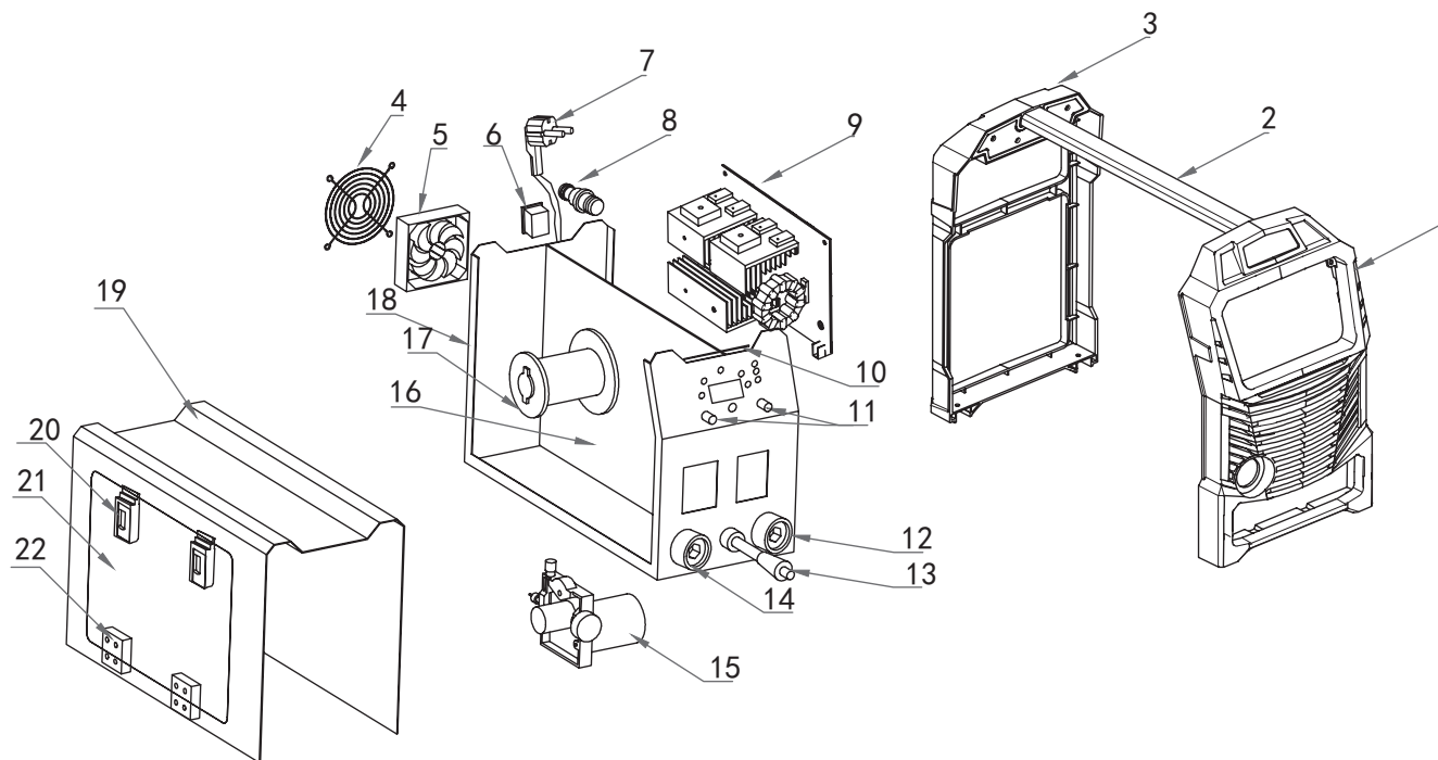
Схема сборки № 1
