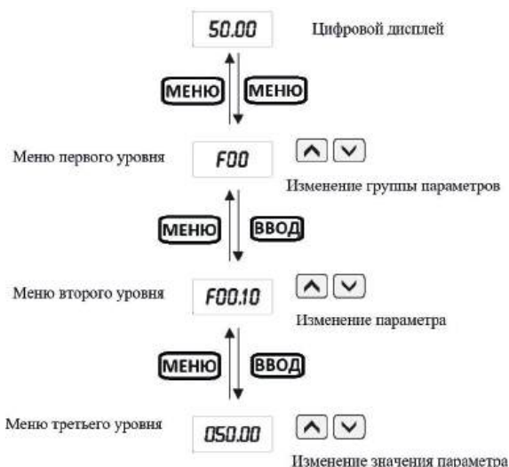
Рис. 6.1 Схема настройки параметров меню
