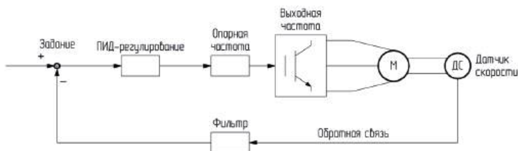
Рис.6.23 Схема ПИД-регулирования
