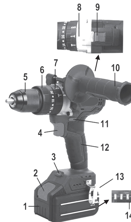
Рис. 1 Общий вид дрели «Redtool» CS-1150Set
