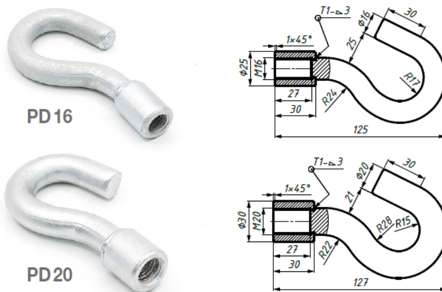
Рис. 1. Внешний вид крюкообразных гаек PD16, PD20.
