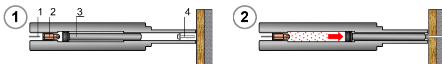
1. Боек. 2. Монтажный патрон. 3. Поршень. 4. Дюбель-гвоздь.
