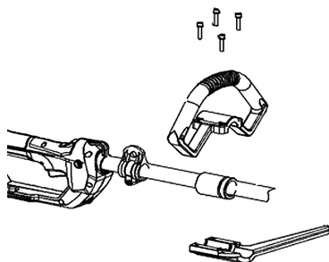
Рис. 4 Установка рукоятки
