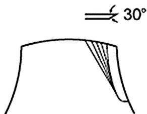
Рис. 11 Заточка ножа
