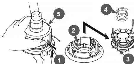
Рис. 17 Разборка триммерной головки
