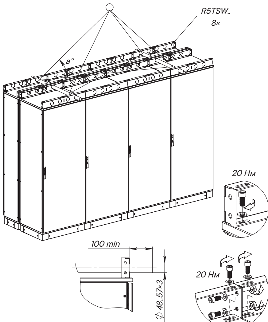
Схема распределения масс шкафов в сборке:
