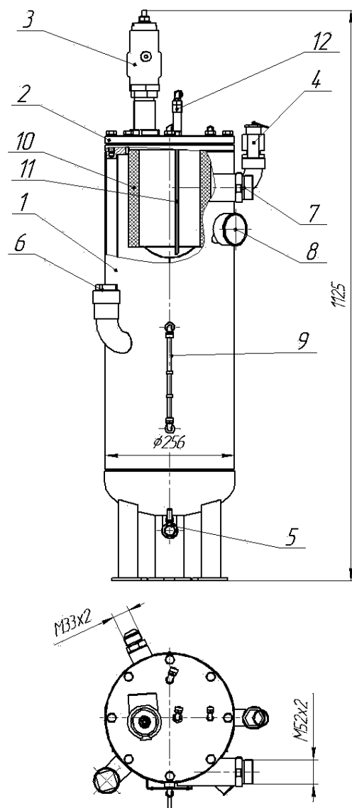
Рисунок 5. Маслоотделитель.
