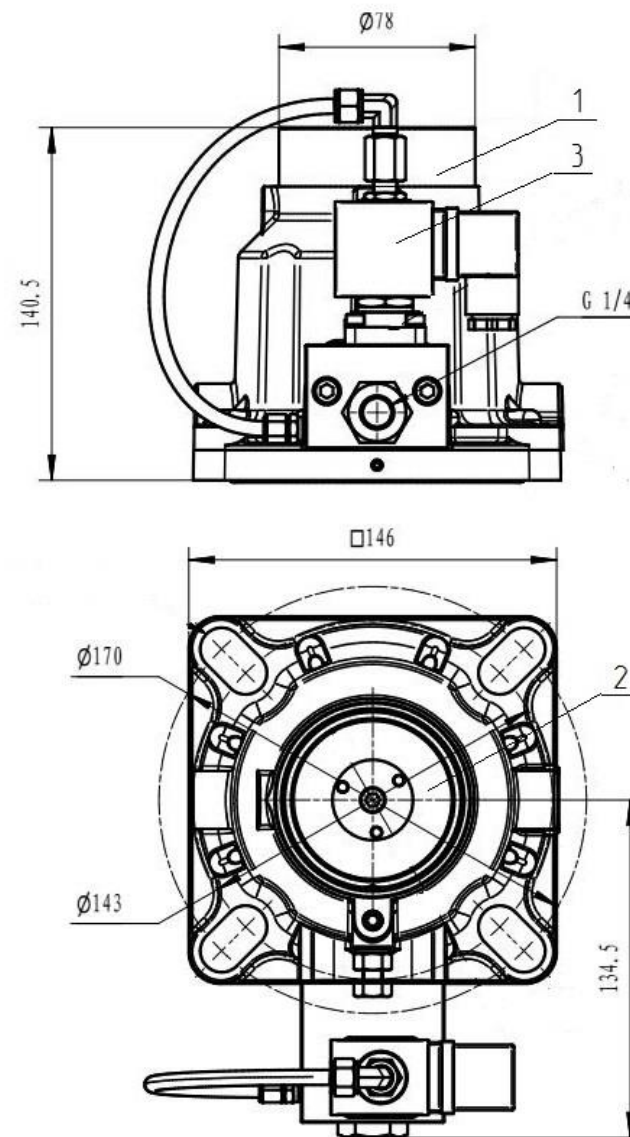
Рисунок 4. Клапан впускной.
