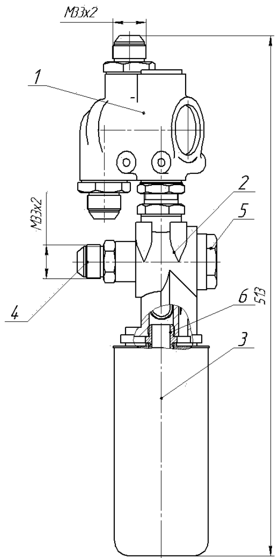
Рисунок 7. Блок распределения.
