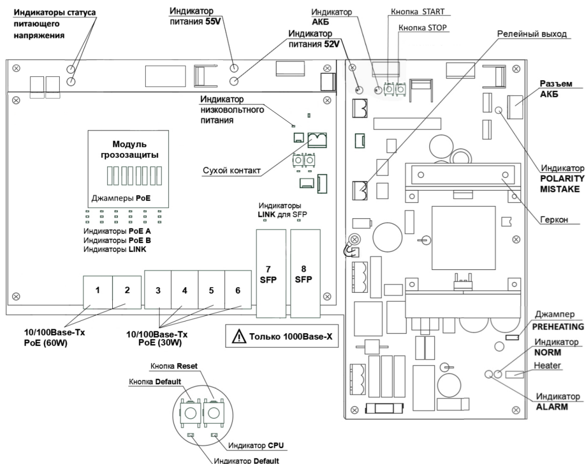
Рисунок 3.4.1 – Расположение элементов PSW-2G6F+UPS-Box
