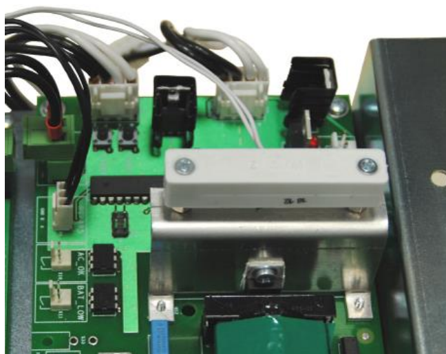
Рисунок 3.7.2 - Датчик вскрытия в корпусе коммутатора
