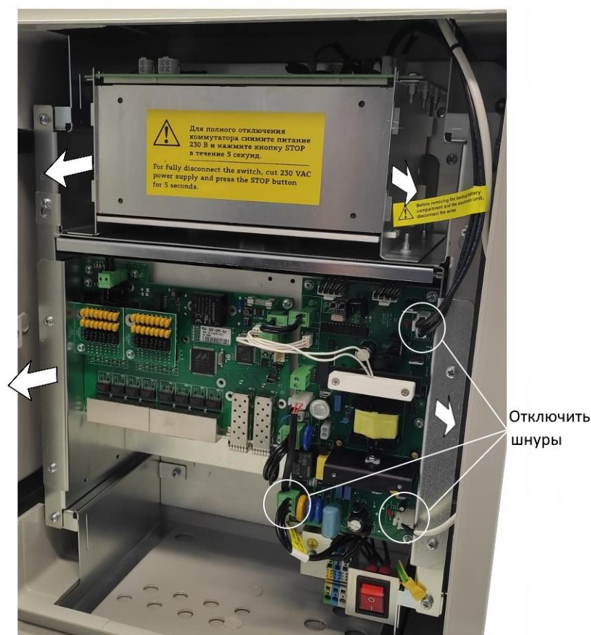
Рис. 7.1.1. Извлечение отсека АКБ и электронного узла
