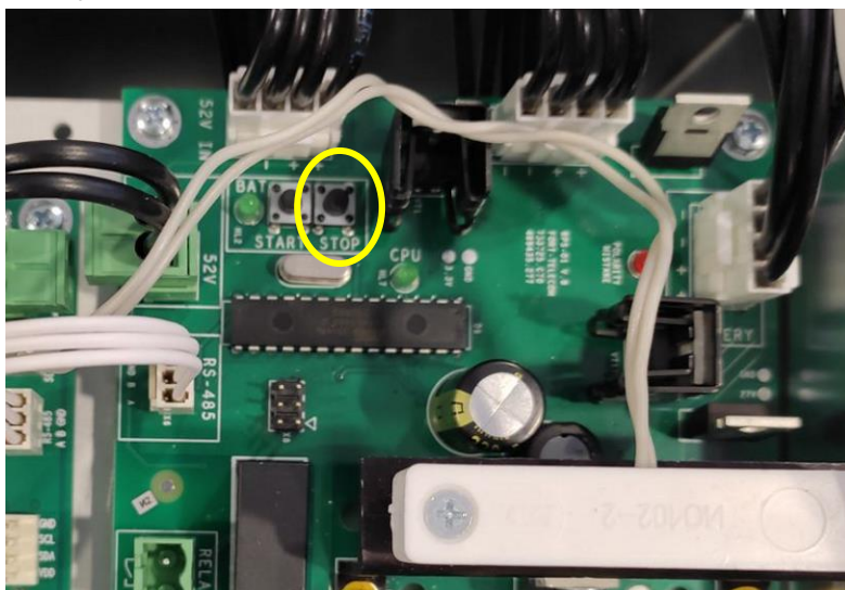
Рисунок 3.5.4 – Нажмите и удерживайте кнопку STOP в течение 5 сек. для отключения питания от АКБ.
