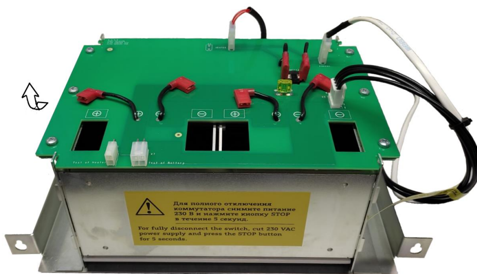
Рисунок 7.6 – Отсек с установленными АКБ.
