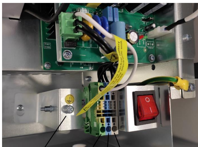
Винт заземления PE N L
