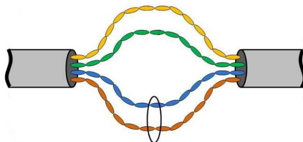
PoE+ «В» (30W)
