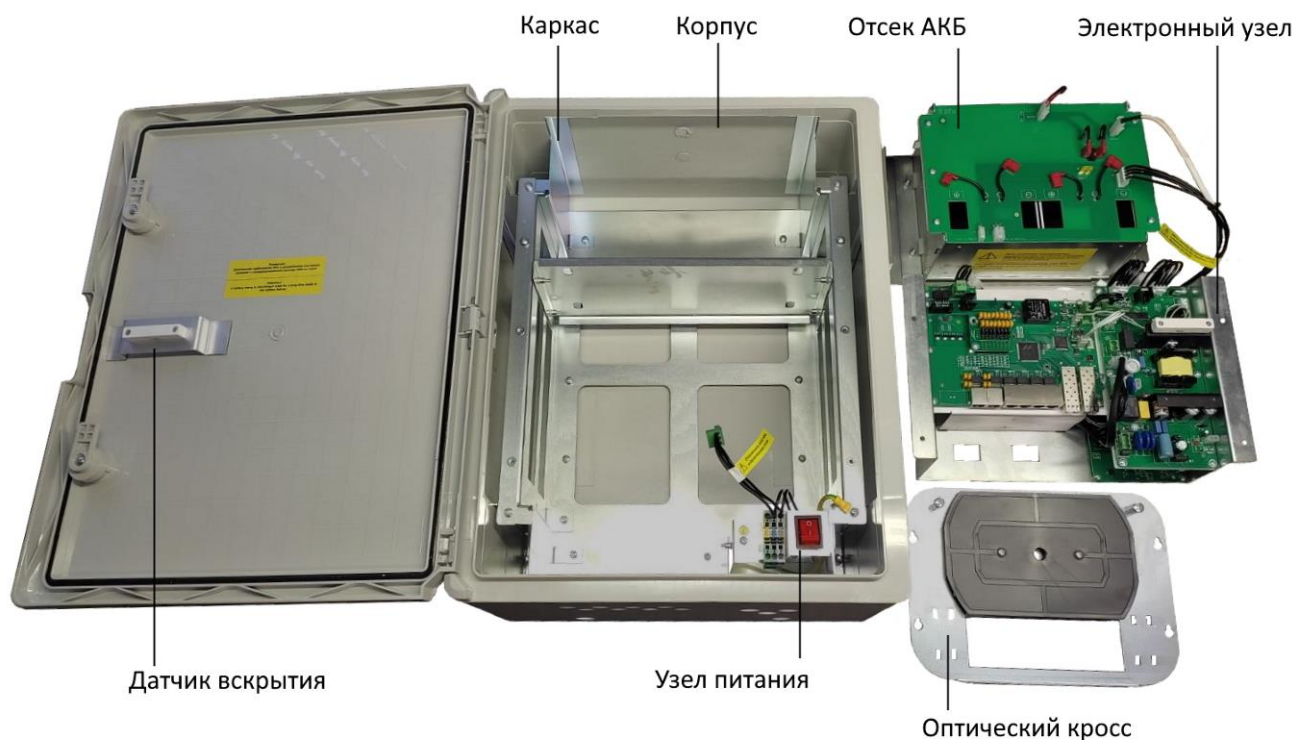
Рисунок 3.1.3 – Основные элементы коммутатора
