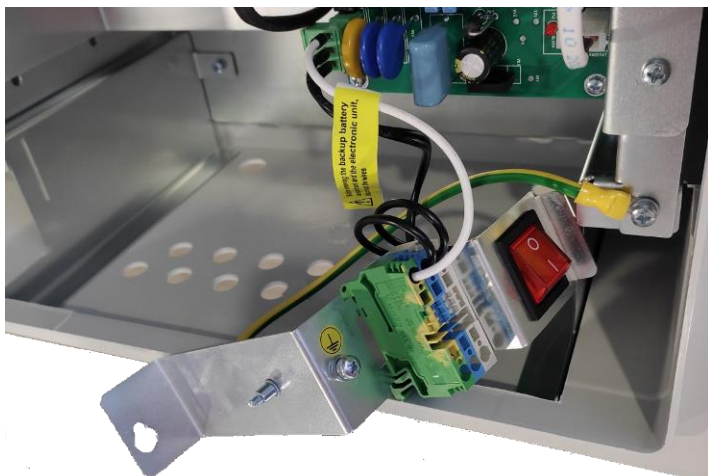
Рисунок 3.5.2 – Узел подключения питания освобожден от крепежа.
