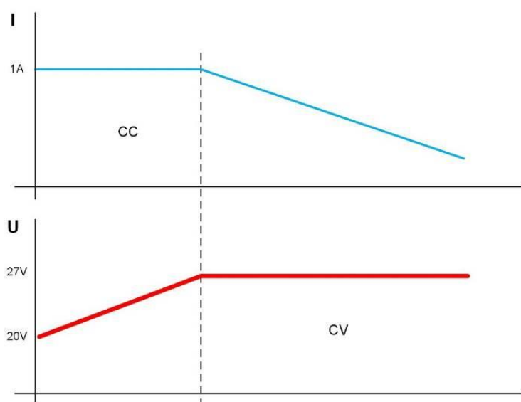
Рисунок 3.11.2 – Зависимость постоянного тока и напряжения заряда АКБ.
