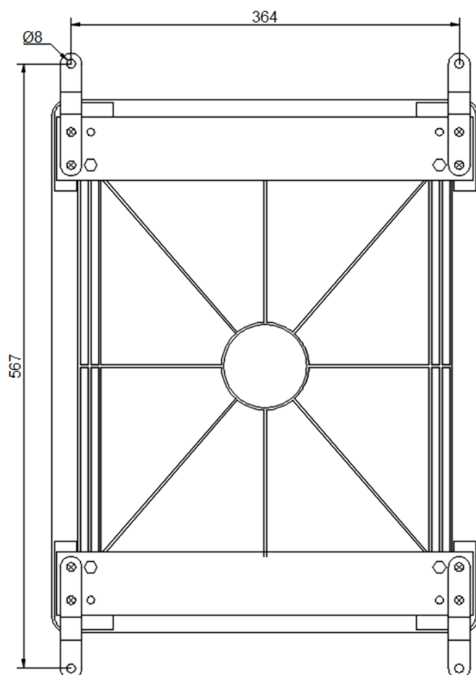
Рисунок 7.2 - Разметка крепления
