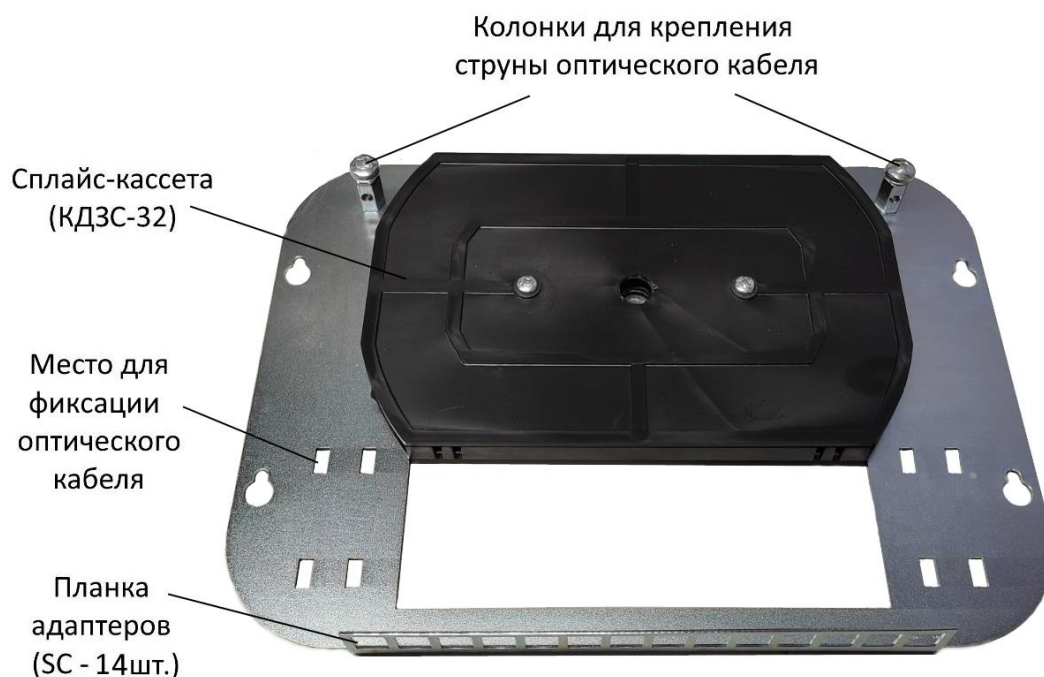
Рисунок 3.3 - Оптический кросс.
