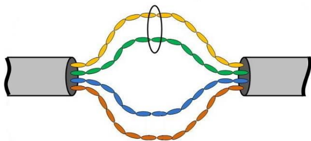
PoE+ «А» (30W)
