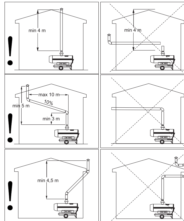
Рисунок 2 — Схема подключения аппарата к дымовой трубе
