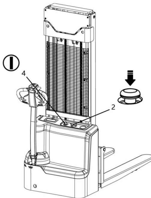
Кнопка подъема/опускания
