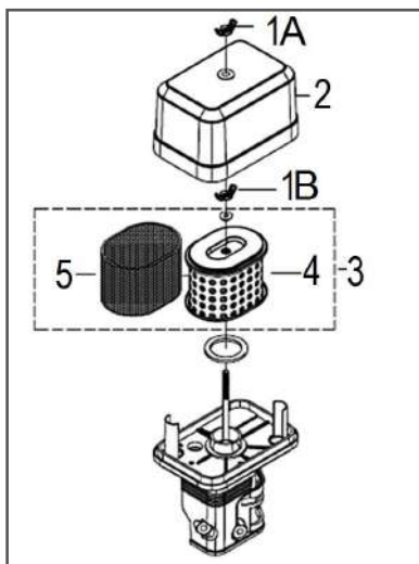
Рис. 35. Обслуживание воздушного фильтра
