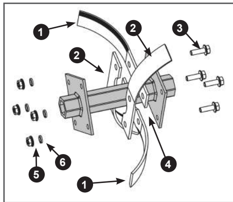
Рис. 17. Установка ножей на внутренний фланец основной секции оси фрезы
