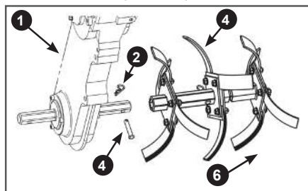
Рис. 21. Установка правой фрезы на вал редуктора
