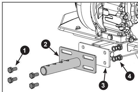
Рис. 13. Установка кронштейна для навесной роторной косилки
