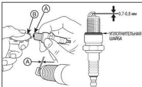
Рис. 39. Проверка межэлектродного зазора А - зазор В - щуп
