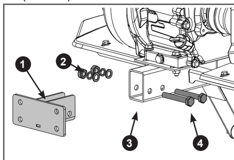
Рис. 12. Установка основания кронштейна для навесной роторной косилки
