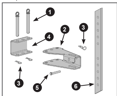
Рис. 7. Установка сошника
