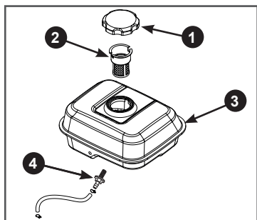
Рис. 36. Топливный бак и топливные фильтры
