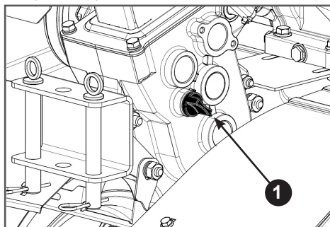
Рис. 26. Крышка маслосазливного отверстия редуктора
