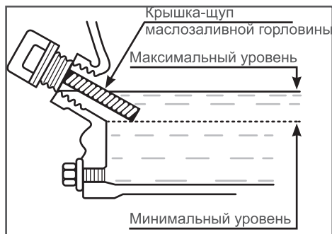
Рис. 24. Проверка уровня масла в картере
