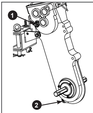
Рис. 40. Замена масла в редукторе
