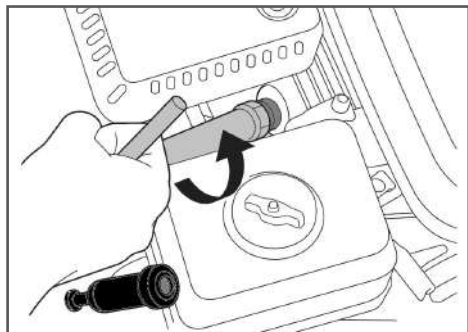
Рис. 38. Обслуживание свечи зажигания
