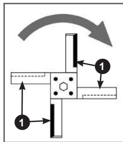
Рис. 15. Расположение ножей на фланцах оси фрезы
