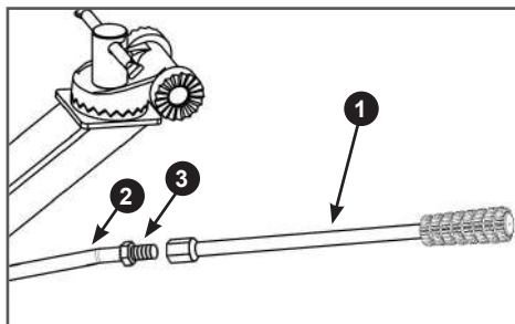
Рис. 10. Установка рычага переключения передач
