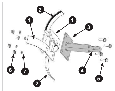
Рис. 19. Сборка дополнительной секции оси фрезы
