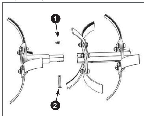
Рис. 20. Соединение основной и дополнительной секций фрезы
