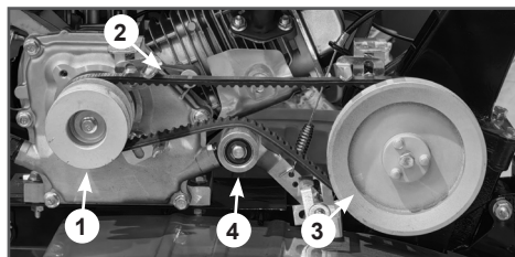
Рис. 41. Замена ремня привода
