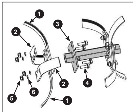
Рис. 18. Установка ножей на внутренний фланец основной секции оси фрезы
