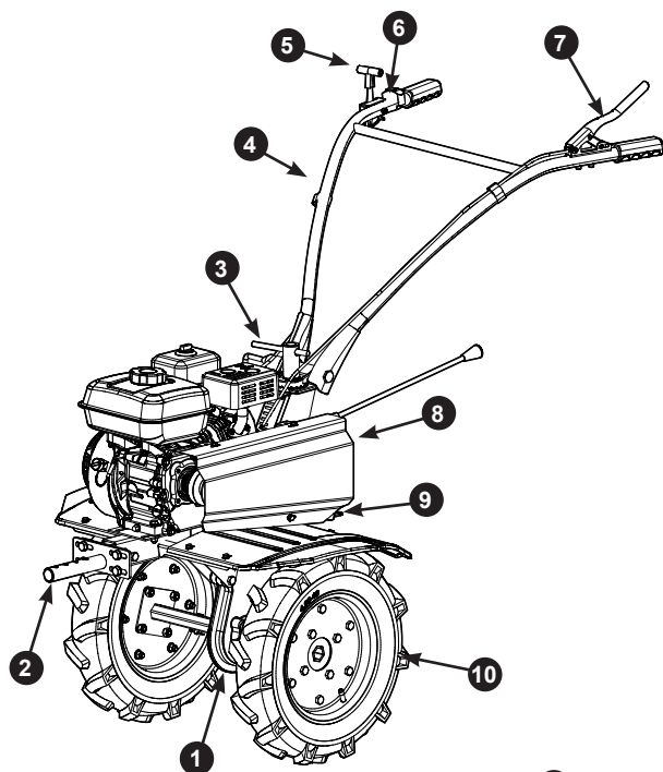
Рис. 1. Основные узлы и органы управления (установлены колёса)
