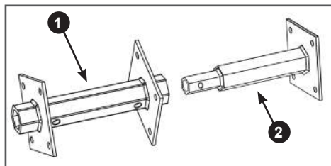
Рис. 16. Секции оси фрезы
