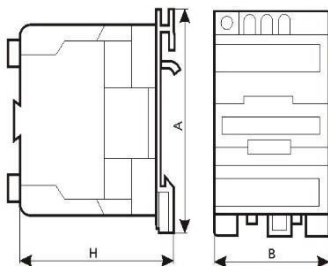
Рисунок 2. Контактор неререверсивный ПМЛ-2
