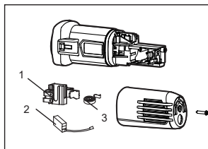
1. Щеткодержатель 2. Угольная щетка 3. Спиральная пружина
