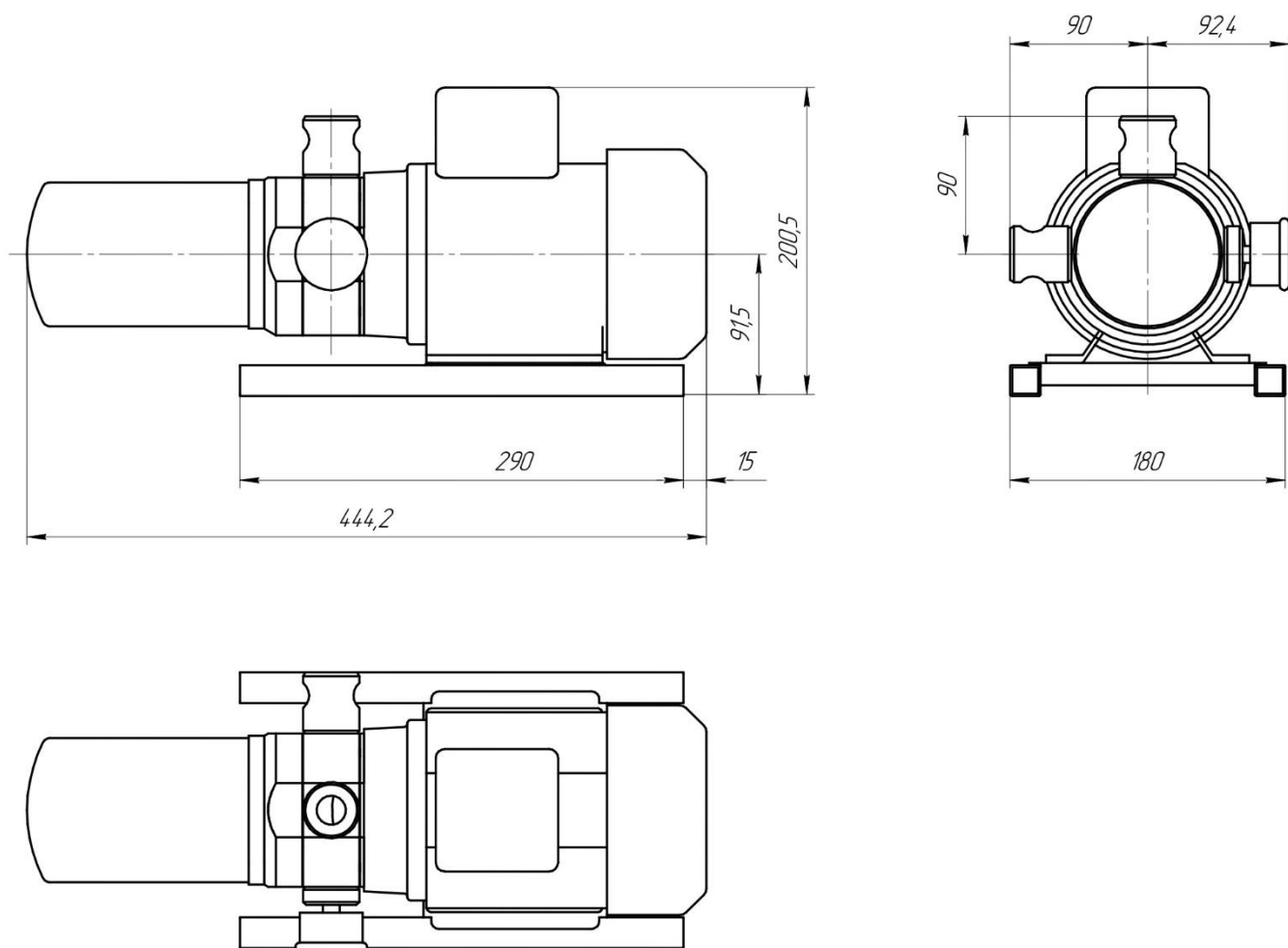
Габаритные размеры
