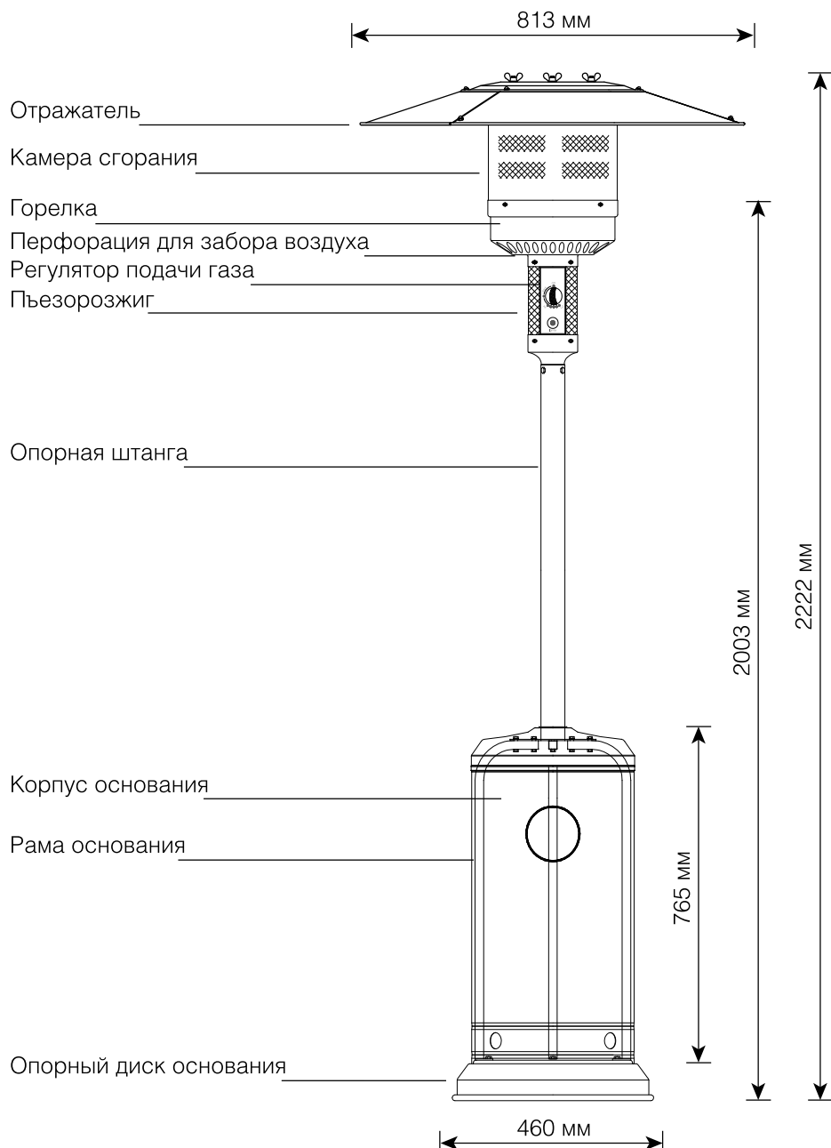
Рис. 2 – устройство модели BOGH Vela.
