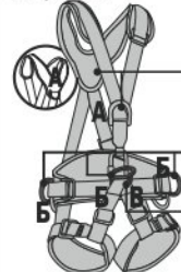
Рис. 4. Расположение и назначение крепежных точек на привязях
