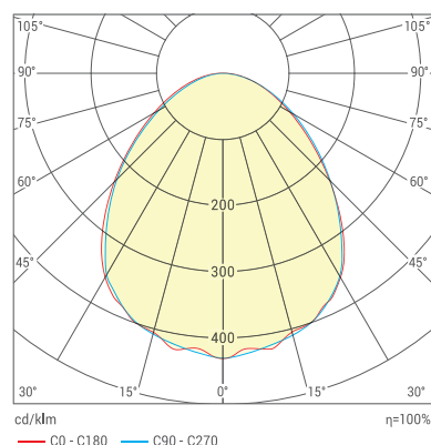
КСС (микропризма)
