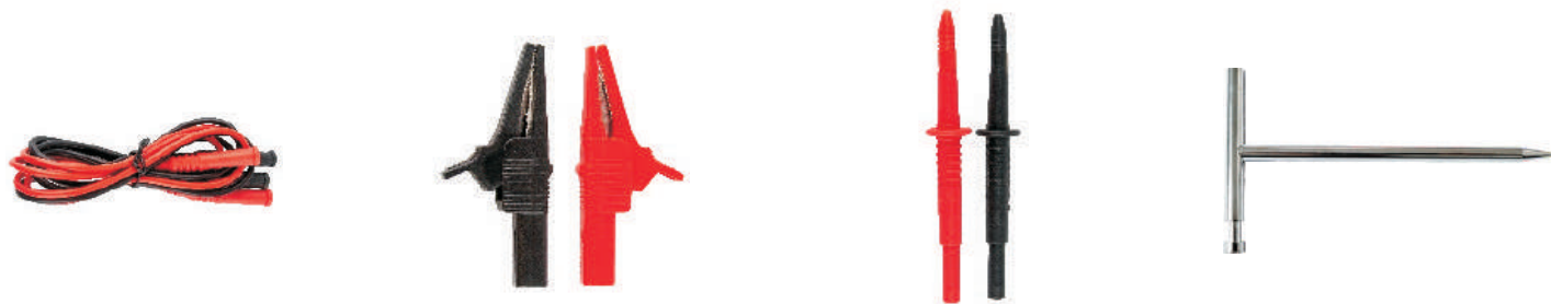
1. Соединительные провода 2. Зажимы типа «крокодил» 3. Измерительные щупы 4. Заземляющий стержень
