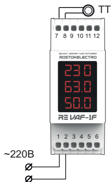
Схема подключения
