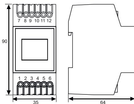
Габаритные размеры
