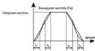
Рис. 6-2 Кривая S разгона/торможения А
