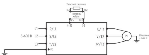
Рис. 3.2.5 Подключение силовых клемм
