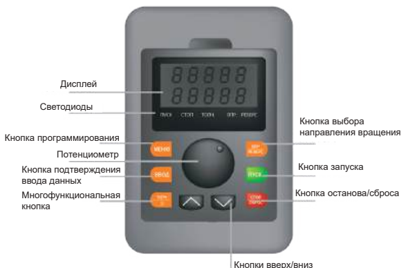
Рис. 5.1 Функции кнопок и светодиодов панели управления LCI
