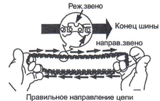
Правильное направление цепи
