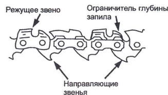
Правильное направление цепи
