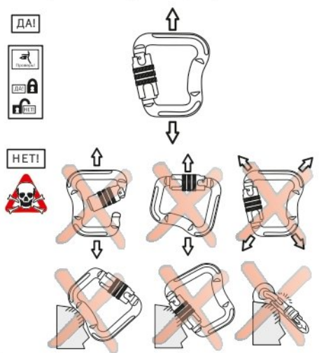
Рис. 3. Приложение нагрузки к карабину
