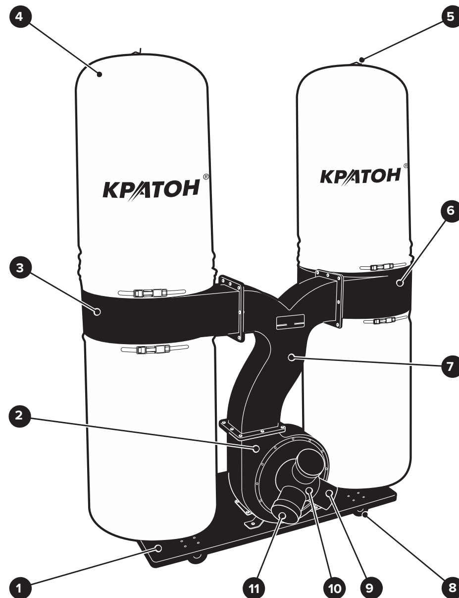
Рисунок 1 — Общий вид пылесоса
