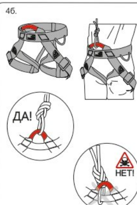
Рис. 5. Подключение страховочных устройств
